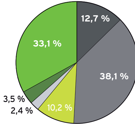
Strom-Mix Deutschland
